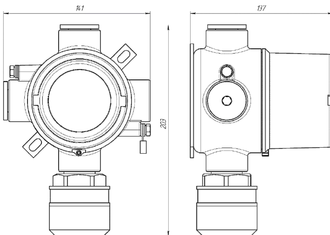
Рисунок 6 – Габаритные размеры ИГМ-11 (корпус тип 3)
