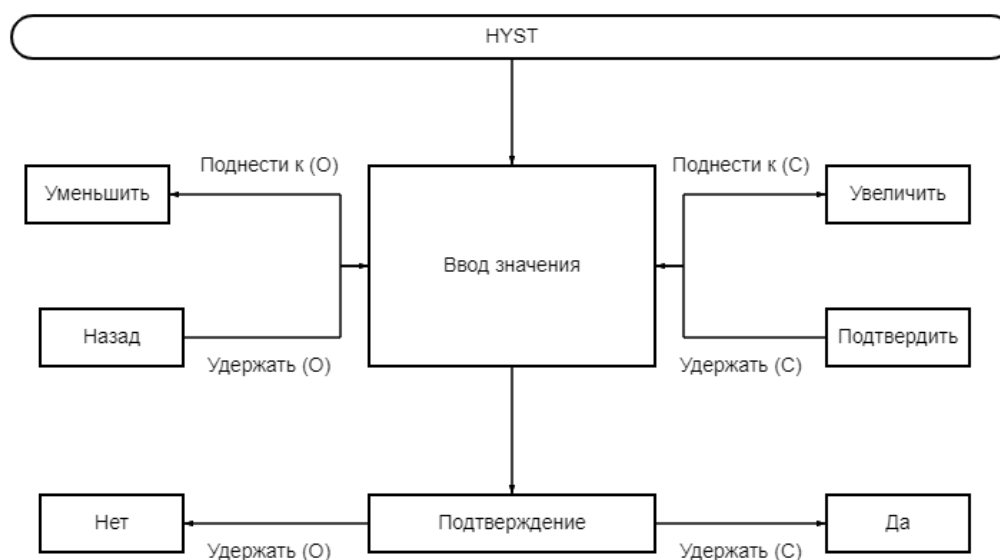
Рисунок К.2.15 – Алгоритм настройки значения гистерезиса
