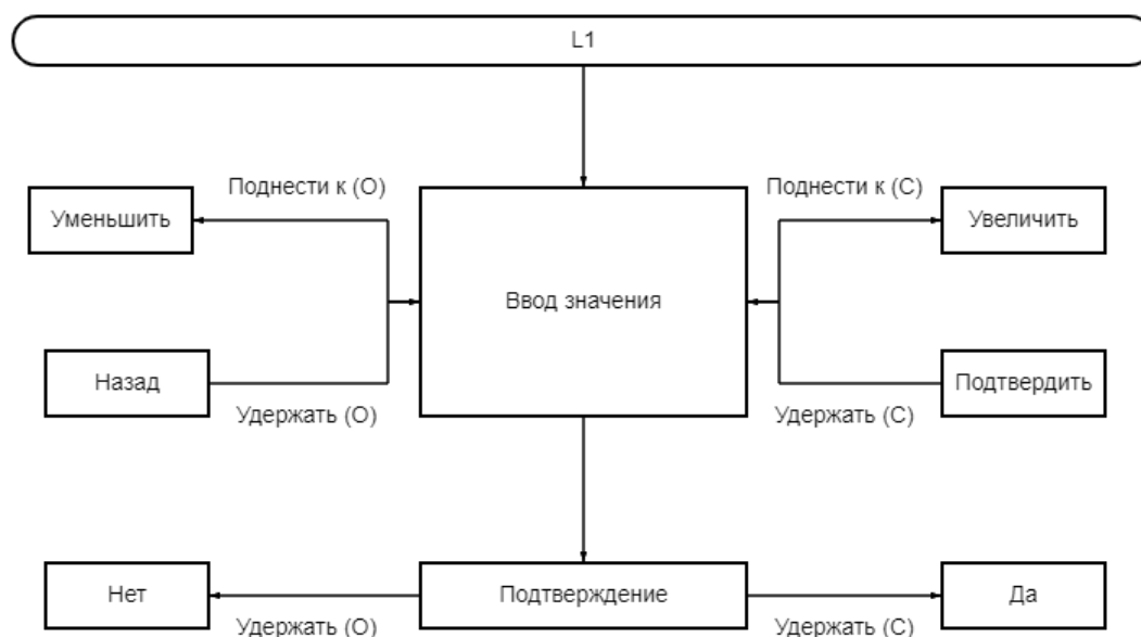
Рисунок К.2.16 – Алгоритм настройки Порога 1
